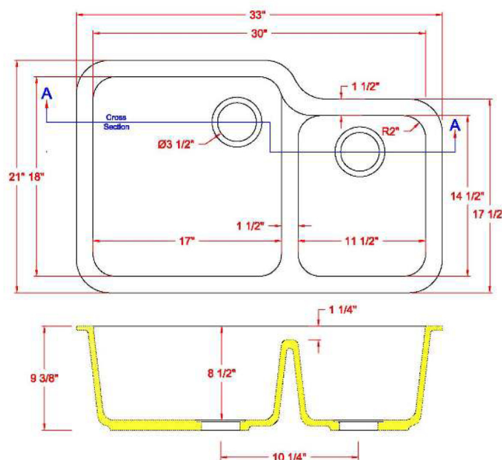
Section A-A 1114-DR
